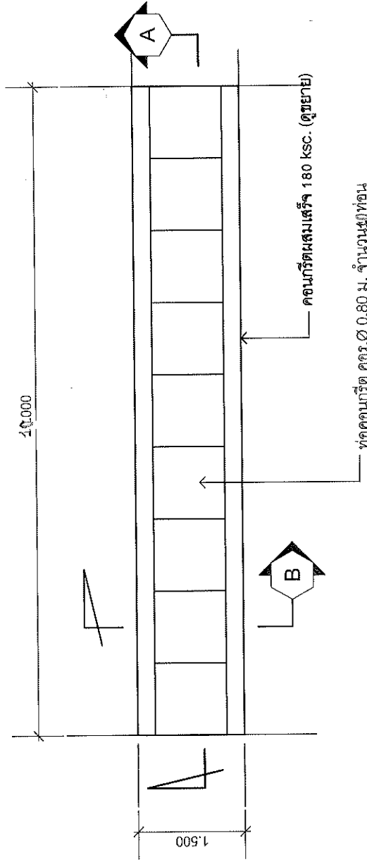
แปลนปรับปรุงวางท่อระบายน้ำคอนกรีต ค.ร. ๓๐.80 ม.
