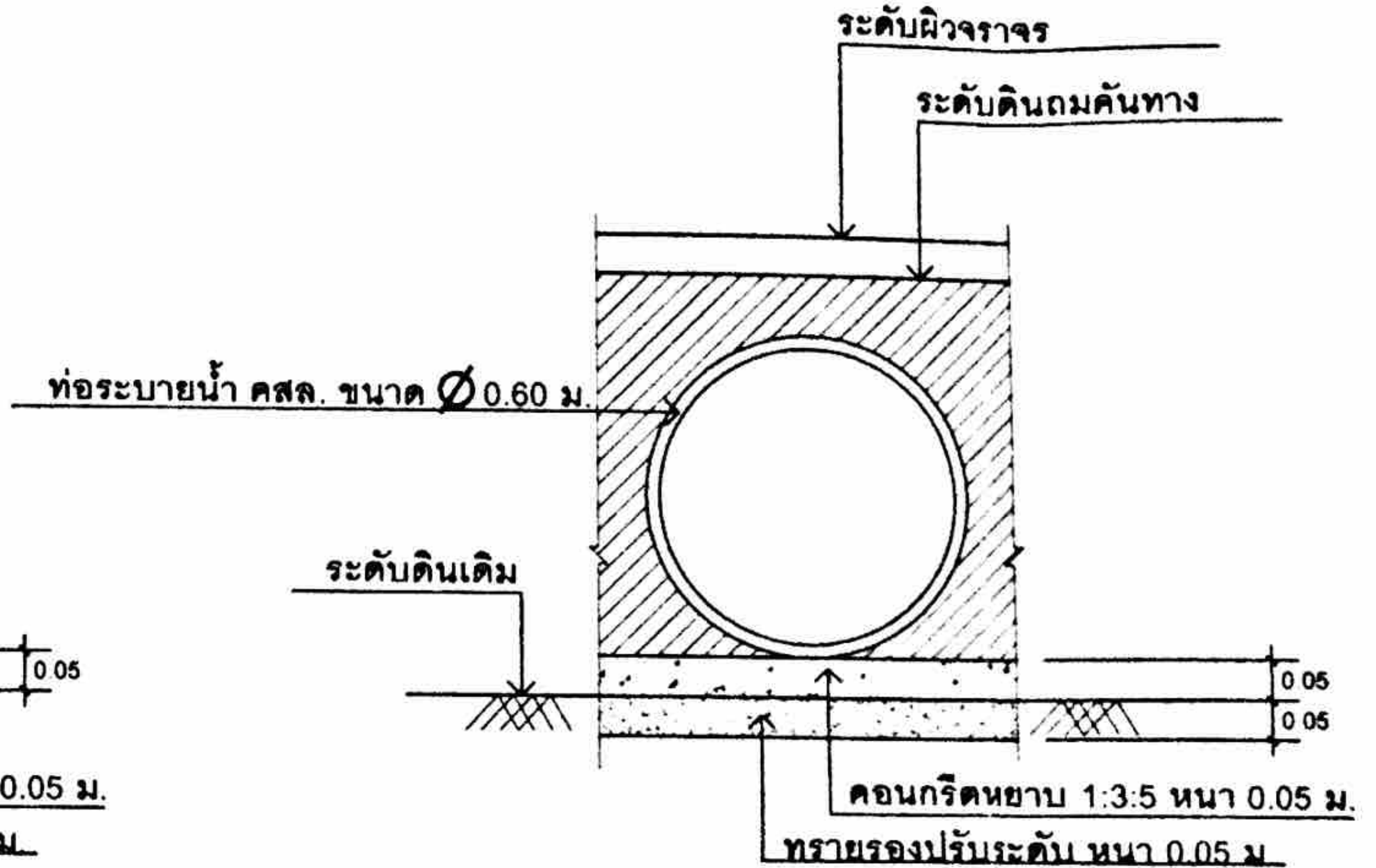
แบบแสดงการวางท่อคอนกรีต ไม่แสดงมาตราส่วน
