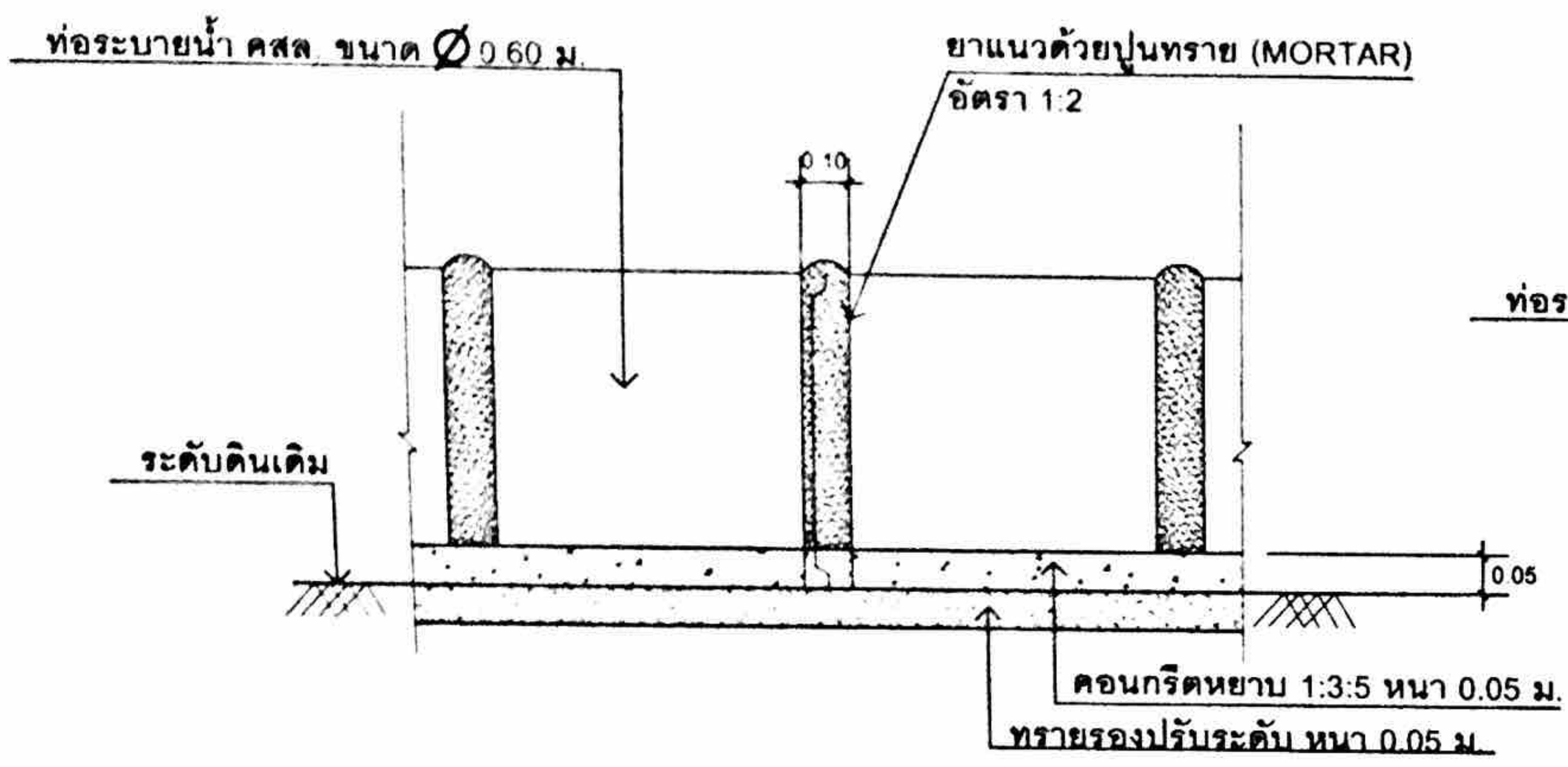
รูปตัดแสดงการต่อท่อยาแนว ไม่แสดงมาตราส่วน
