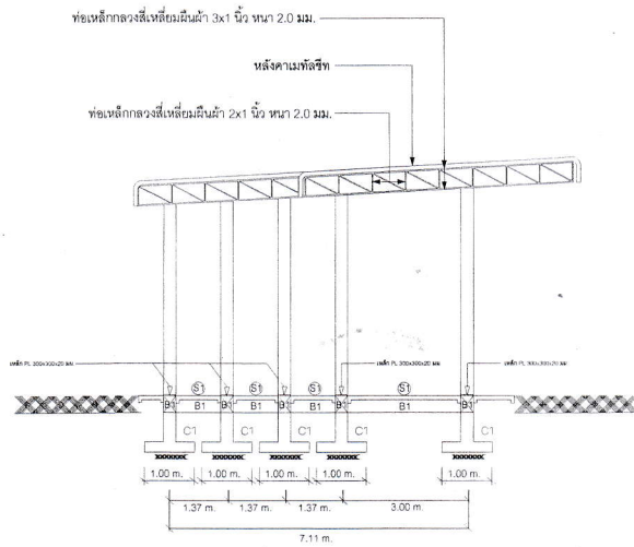
รูปด้าน ข 1:100
