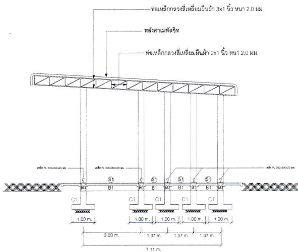
รูปด้าน ก 1:100
