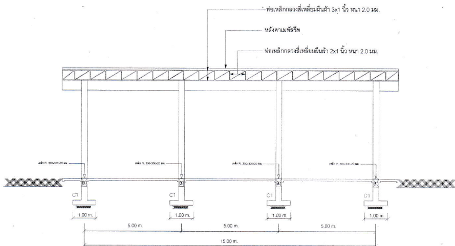
รูปด้าน ด 1:100
